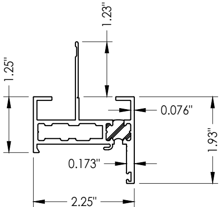
6 FIN BLOCK FRAME
