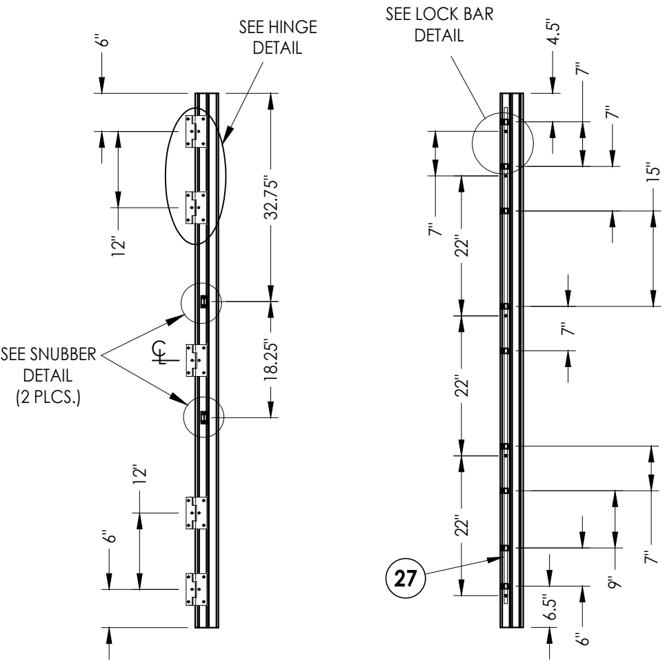
HINGE JAMB
